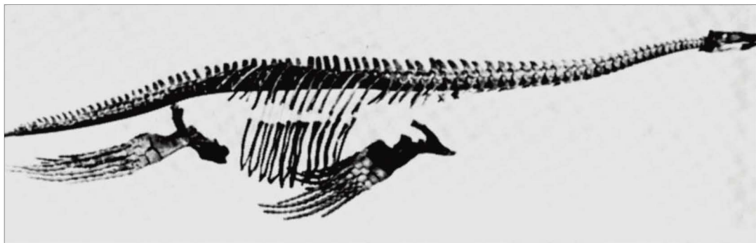
Brancasaurus brancai Wegner, vrijwel compleet skelet, afkomstig uit de voormalige groeve Gerdemann, Gronau, in het Geologisch Instituut te Münster.
