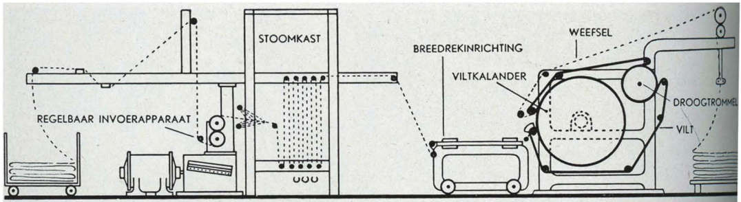
Doorsnede sanforiseermachine.
