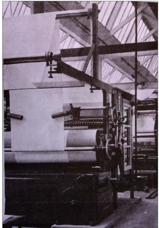
De eerste Sanforiseermachine bij de Nederlandsche Stoomblekerij Nijverdal, ca. 1947.
