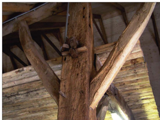
Detailfoto van de ankerbalkconstructie. Op de gebintstijl en op de twee schoren (of korbelen) zijn telmerken zichtbaar. Gebinten werden eerst op maat gemaakt en vervolgens, op de plek van bestemming, in elkaar gezet.
